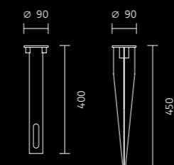
Erdanker und Erdspieß / Ground anchor and ground spike
