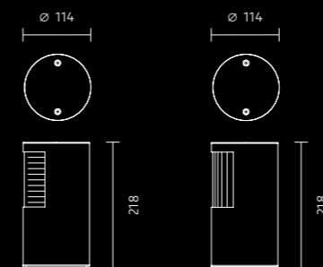
Horizontallamellen / Horizontal louvres
