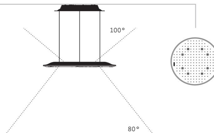
Abstrahlwinkel
